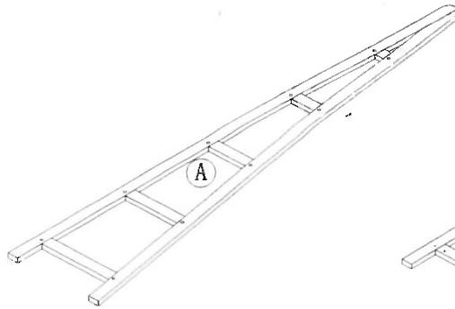
A. LEFT SIDE FRAME 1PC
